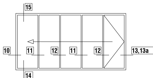
INWARD OPENING 5 PANELS ON ONE SIDE FOLDING DOOR ΕΞΩ ΑΝΟΙΓΟΜΕΝΗ 5 ΦΥΛΛΗ ΦΥΣΟΥΝΑ ΣΕ ΜΙΑ ΠΛΕΥΡΑ
