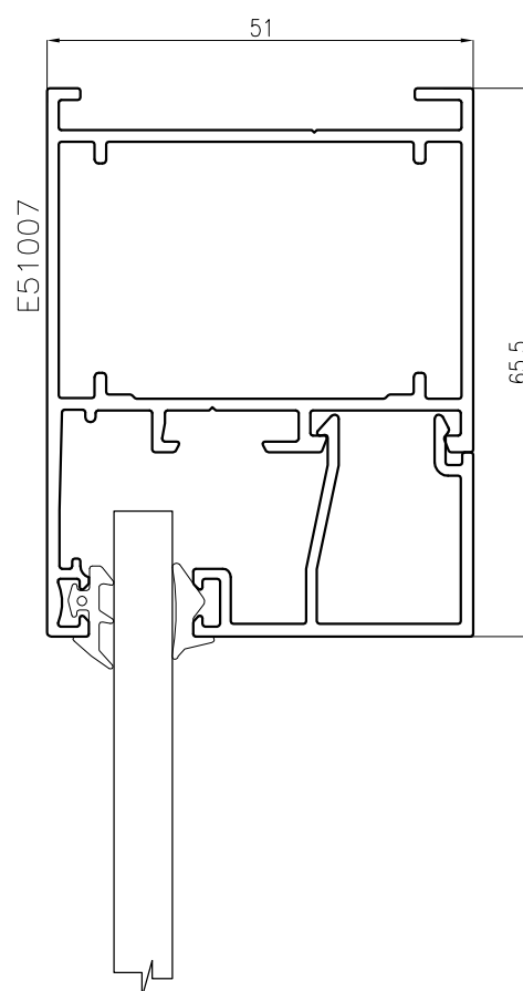
SEZIONE 10
