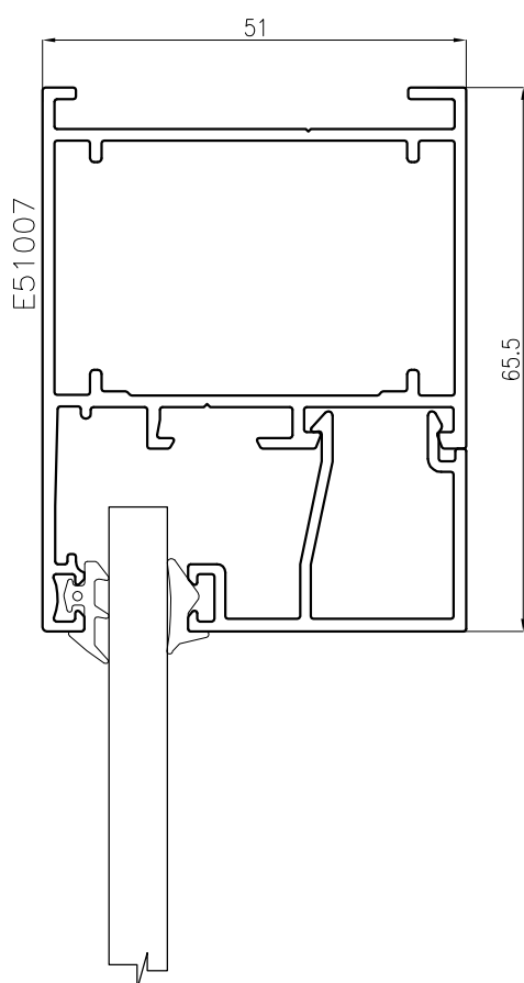
SEZIONE 2
