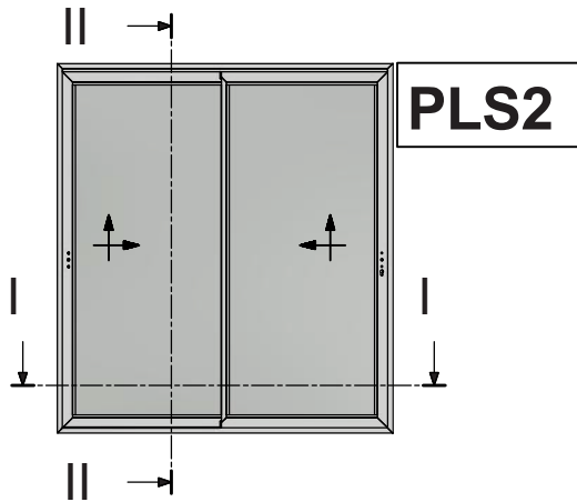
Two Sash Parallel Lift & Slide Window with Narrow Interlock use only S560 Δίφυλλο Επάλληλο Ανασυρόμενο με Στενό Γάντζο με χρήση μόνο μικρού φύλλου S560
