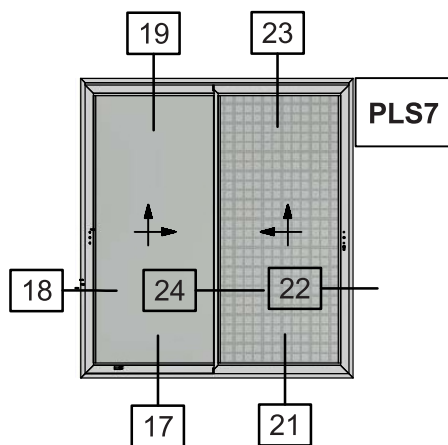
Two Sash Parallel with Narrow Interlock and Flyscreen Lift & Slide Window S560 sash use only Δίφυλλο Επάλληλο Ανασυσρόμενο με Στενό Γάντζο και Σήτα με χρήση φύλλου S560
