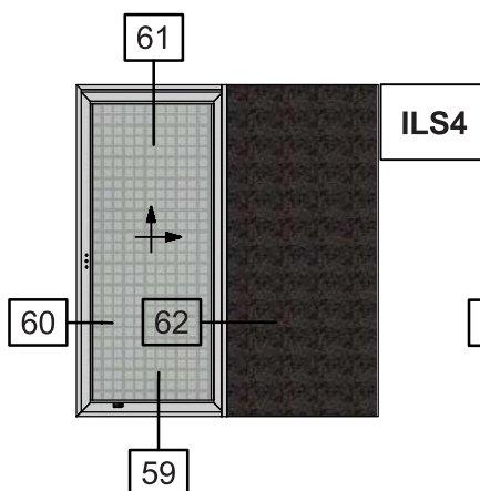
Single Sash Pocket Lift & Slide Window with Flyscreen and Shutter Short sash use only S560 Μονόφυλλο Χωνευτό Ανασπώμενο με Σήτα και Παντζούρι με χρήση μικρού φύλλου S560
