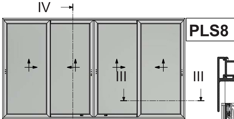
Four Sash Parallel Meeting Stile Lift & Slide Window S560 sash use only Τετράφυλλο Επάλληλο Φιλητό Ανασυρόμενο με χρήση φύλλου S560
