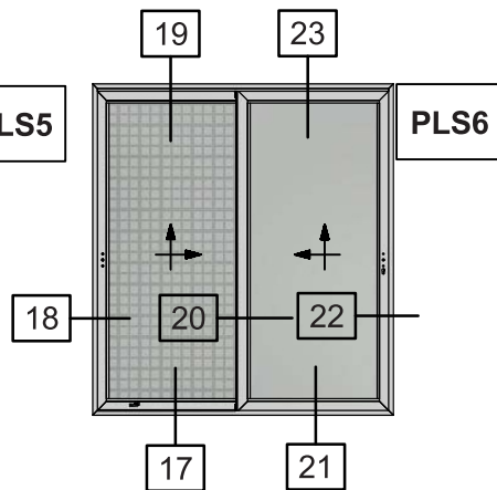
Two Sash Parallel with Flyscreen Lift & Slide Window S560 sash use only Δίφυλλο Επάλληλο Ανασυσρόμενο με Σήτα με χρήση φύλλου S560
