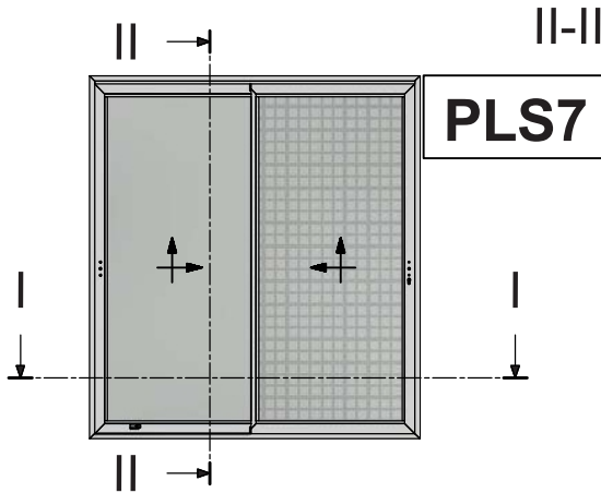
Two Sash Parallel with Narrow Interlock and Flyscreen Lift & Slide Window S560 sash use only Δίφυλλο Επάλληλο Ανασυσρόμενο με Στενό Γάντζο και Σήτα με χρήση φύλλου S560
