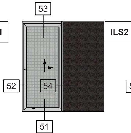
Single Sash Pocket Lift & Slide Window with Flyscreen Short sash use only S560 Μονόφυλλο Χωνευτό Ανασπώμενο με Σήτα με χρήση μικρού φύλλου S560
