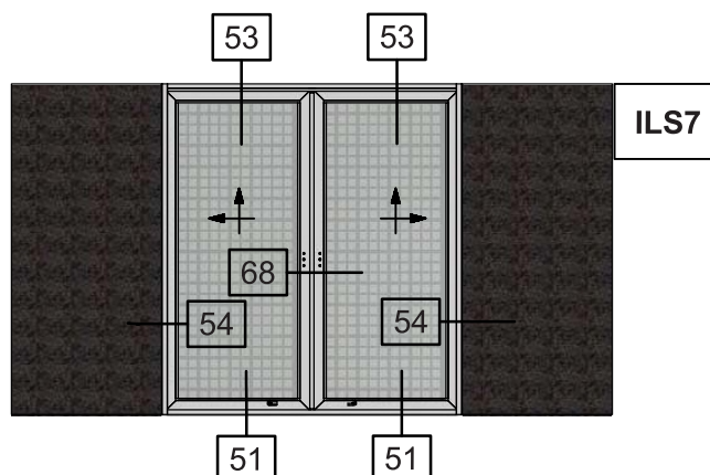
Two Sash Meeting Stile Pocket Lift & Slide Window with Flyscreen Short sash use only S560 Δίφυλλο Φιλητό Χωνευτό Ανασυρόμενο με Σήτα με χρήση μικρού φύλλου S560
