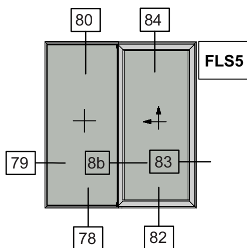
Fixed - Lift & Slide Window with Fixed on the Outside Narrow Interlock Σταθερό - Ανασυρόμενο με το Σταθερό Εξωτερικά με στενό γάντζο
