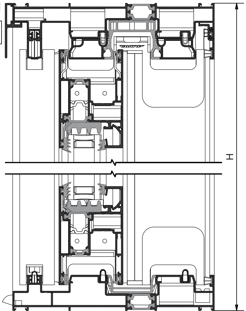
Two Sash Parallel with Narrow Interlock and Flyscreen Lift & Slide Window S560 sash use only Δίφυλλο Επάλληλο Ανασυσρόμενο με Στενό Γάντζο και Σήτα με χρήση φύλλου S560
