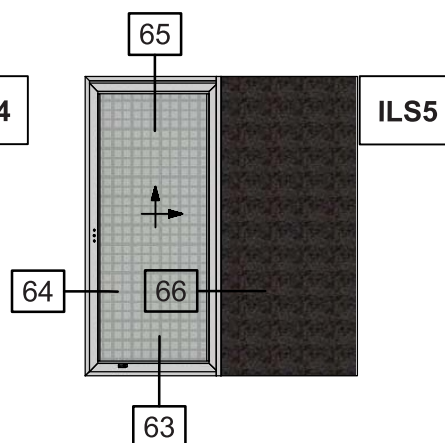
Single Sash Pocket Lift & Slide Window with Narrow Flyscreen and Shutter Short sash use only S560 Μονόφυλλο Χωνευτό Ανασπώμενο με Στενή Σήτα και Παντζούρι με χρήση μικρού φύλλου S560
