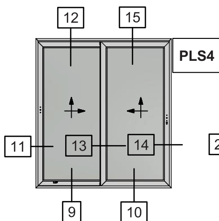
Two Sash Parallel Lift & Slide Window Large sash use only S584 Δίφυλλο Επάλληλο Ανασυσρόμενο με χρήση μεγάλου φύλλου S584
