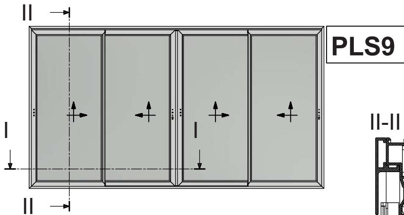
Four Sash Parallel Meeting Stile with Narrow Interlock Lift & Side Window S560 sash use only Τετράφυλλο Επάλληλο Φιλητό Ανασυρόμενο με Στενό Γάντζο με χρήση φύλλου S560
