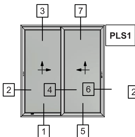
Two Sash Parallel Lift & Slide Window Short sash use only S560 Δίφυλλο Επάλληλο Ανασυσρόμενο με χρήση μικρού φύλλου S560
