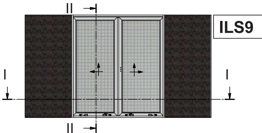
Δίφυλλο Φιλητό Χωνευτό Ανασυρόμενο με Στενή Σήτα και Παντζούρι με χρήση μικρού φύλλου S560 Two Sash Meeting Stile Pocket Lift & Slide Window with Narrow Flyscreen and Shutter Short sash use only S560
