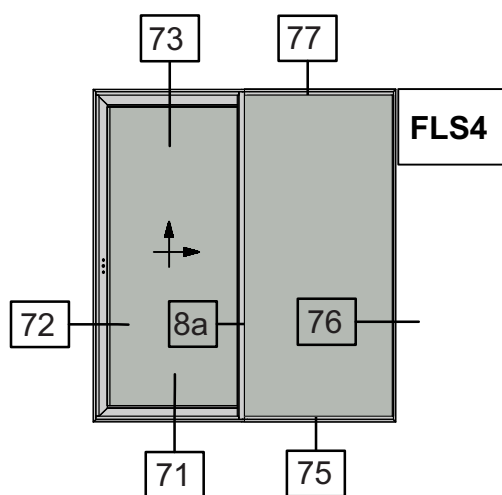
Fixed - Lift & Slide Window with Fixed on the Inside Narrow Interlock Σταθερό - Ανασυρόμενο με το Σταθερό Εσωτερικά με στενό γάντζο
