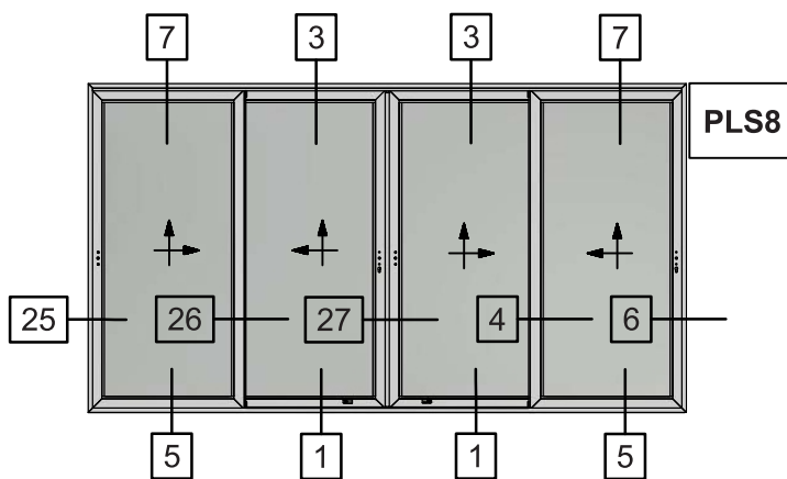
Four Sash Parallel Meeting Stile Lift & Slide Window S560 sash use only Τετράφυλλο Επάλληλο Φιλητό Ανασυσρόμενο με χρήση φύλλου S560
