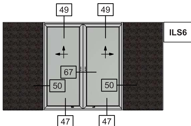
Two Sash Meeting Stile Pocket Lift & Slide Window Short sash use only S560 Δίφυλλο Φιλητό Χωνευτό Ανασυρόμενο με χρήση μικρού φύλλου S560
