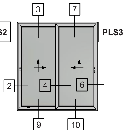
Two Sash Parallel Lift & Slide Window using S560-S584 Δίφυλλο Επάλληλο Ανασυσρόμενο με τη χρήση S560-S584
