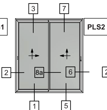
Two Sash Parallel Lift & Slide Window with Narrow Interlock Δίφυλλο Επάλληλο Ανασυσρόμενο με Στενό Γάντζο
