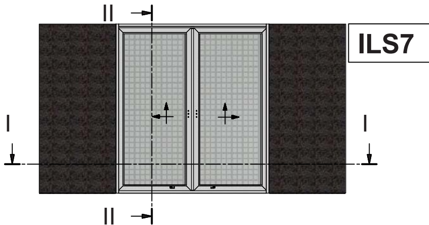
Two Sash Meeting Stile Pocket Lift & Slide Window with Flyscreen Short sash use only S560 Δίφυλλο Φιλητό Χωνευτό Ανασπρόμενο με Σήτα με χρήση μικρού φύλλου S560
