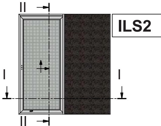
Single Sash Pocket Lift & Slide Window with Flyscreen Short sash use only S560 Μονόφυλλο Χωνευτό Ανασυρόμενο με Σήτα με χρήση μικρού φύλλου S560
