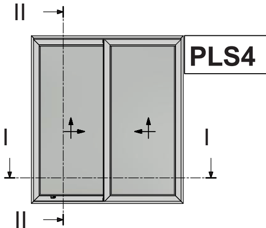
Two Sash Parallel Lift & Slide Window large sash use only S584 Δίφυλλο Επάλληλο Ανασπώμενο με χρήση μεγάλου φύλλου S584
