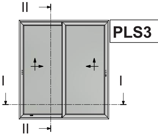
Two Sash Parallel Lift & Slide Window using S560-S584 Δίφυλλο Επάλληλο Ανασυσρόμενο με τη χρήση S560-S584
