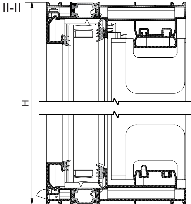
Fixed - Lift & Slide Window with Fixed on the Outside Narrow Interlock Σταθερό - Ανασπώμενο με το Σταθερό Εξωτερικά με στενό γάντζο
