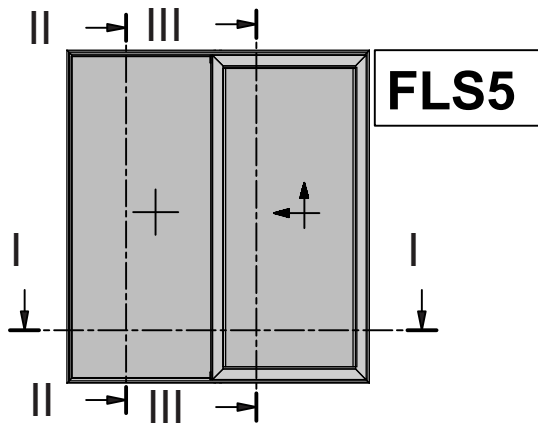
Fixed - Lift & Slide Window with Fixed on the Outside Narrow Interlock Σταθερό - Ανασπώμενο με το Σταθερό Εξωτερικά με στενό γάντζο
