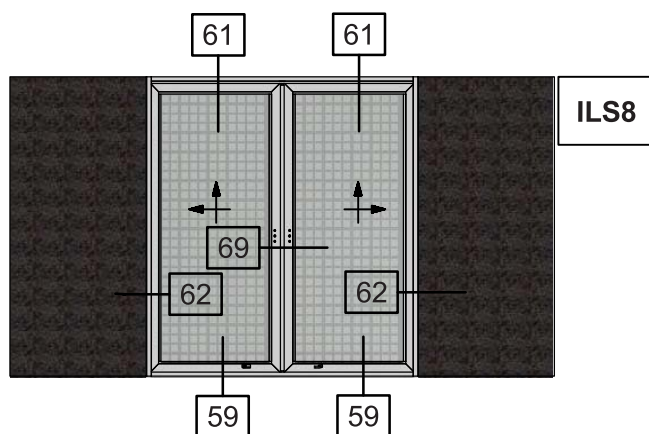
Two Sash Meeting Stile Pocket Lift & Slide Window with Flyscreen and Shutter Short sash use only S560 Δίφυλλο Φιλητό Χωνευτό Ανασυρόμενο με Σήτα και Παντζούρι με χρήση μικρού φύλλου S560
