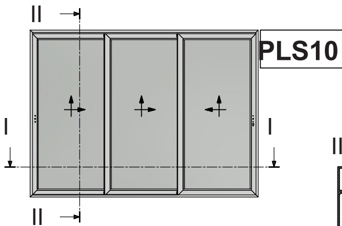
Three Sash Parallel Lift & Slide Window S560 sash use only Τρίφυλλο Επάλληλο Ανασυρόμενο με χρήση φύλλου S560
