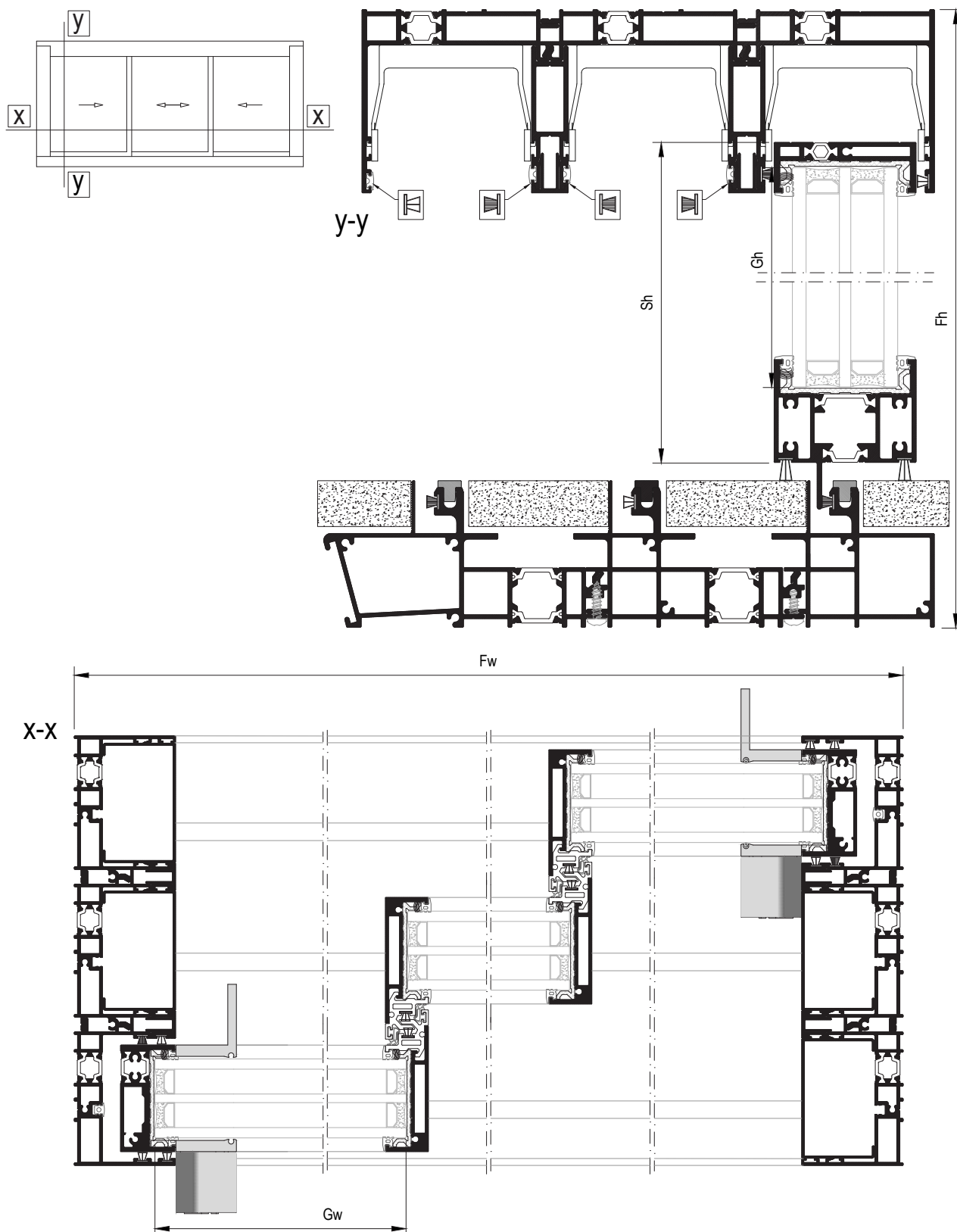
C Three-sash parallel sliding window Τρίφυλλο επάλληλο συρόμενο
