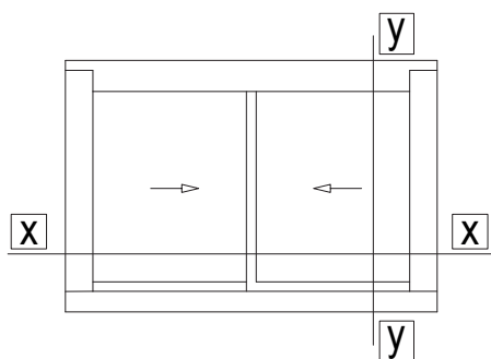
A Two-sash sliding window Δίφυλλο επάλληλο συρόμενο
