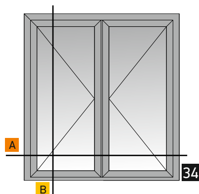
Double side-hung door inward opening without threshold Δίφυλλη πόρτα ανοιγόμενη μέσα με λάστιχο χωρίς κατωκάσι
