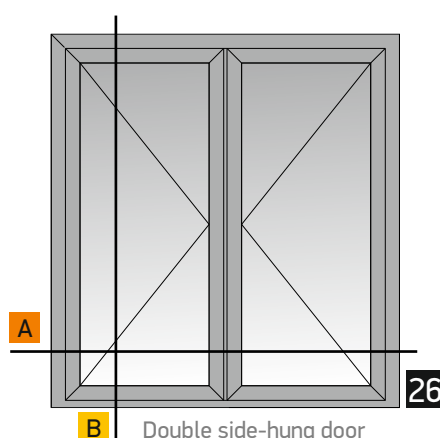
Double side-hung door inward opening without threshold Δίφυλλη πόρτα ανοιγόμενη μέσα με πλαστικό χωρίς κατωκάσι
