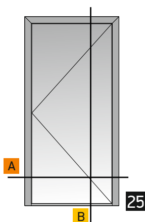
Single leaf door inward opening Μονόφυλλη πόρτα ανοιγόμενη μέσα με πλαστικό χωρίς κατωκάσι
