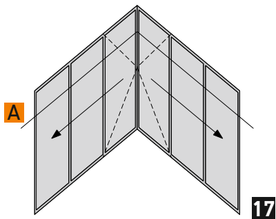
3+3 CORNER TYPOLOGY OUTWARD OPENING 3+3 ΓΩΝΙΑΚΗ ΤΥΠΟΛΟΓΙΑ ΕΞΩ ΑΝΟΙΓΟΜΕΝΗ
