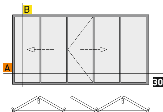
OUTWARD OPENING 3+ 2 PANELS FOLDING DOOR ΕΞΩ ΑΝΟΙΓΟΜΕΝΗ 3+2 5 ΦΥΛΛΗ ΦΥΣΟΥΝΑ
