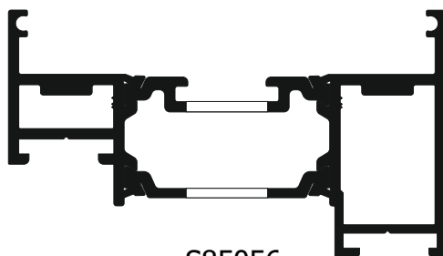
S85056 DOOR ADJUSTER PROFILE
