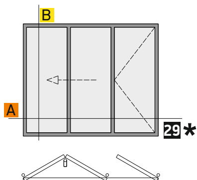
STRUCTURAL OUTWARD OPENING 2+1 3-PANELS FOLDING DOOR LOW THRESHOLD ΗΜΙΔΟΜΙΚΗ ΕΞΩ ΑΝΟΙΓΟΜΕΝΗ 2+1 3-ΦΥΛΛΗ ΦΥΣΟΥΝΑ ΧΑΜΗΛΟ ΚΑΤΩΚΑΣΙ
