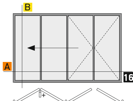
SEMI-STRUCTURAL OUTWARD OPENING, 3+1 4-PANELS FOLDING DOOR STANDARD THRESHOLD ΗΜΙΔΟΜΙΚΗ ΕΞΩ ΑΝΟΙΓΟΜΕΝΗ, 3+1 4-ΦΥΛΛΗ ΦΥΣΟΥΝΑ ΚΑΝΟΝΙΚΟΣ ΟΔΗΓΟΣ
